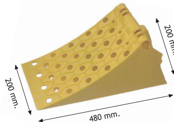
Cod. 95805 Zoccolo / Wheel chock Cod. 95806 Zoccolo + supporto Wheel chock + holder
