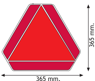
Cod. 70070 RF Segnale in alluminio per veicoli agricoli lenti Aluminium markerboard for slow moving vehicles
