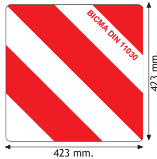
Pannello fisso zincato con angoli arrotondati 423x423 ± 0,8 mm. Panel zinc plated with rounded corners 423x423 ± 0,8 mm.
