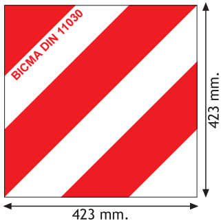
Pannello fisso zincato 423x423 ± 0,8 mm. Panel zinc plated 423x423 ± 0,8 mm.
