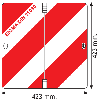
Pannello pieghevole in verticale zincato con angoli arrotondati 423x423 ± 0,8 mm. Vertical folding panel zinc plated with rounded corners 423x423 ± 0,8 mm.
